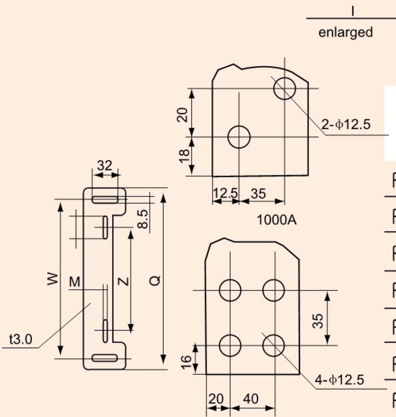
1250~1600A
